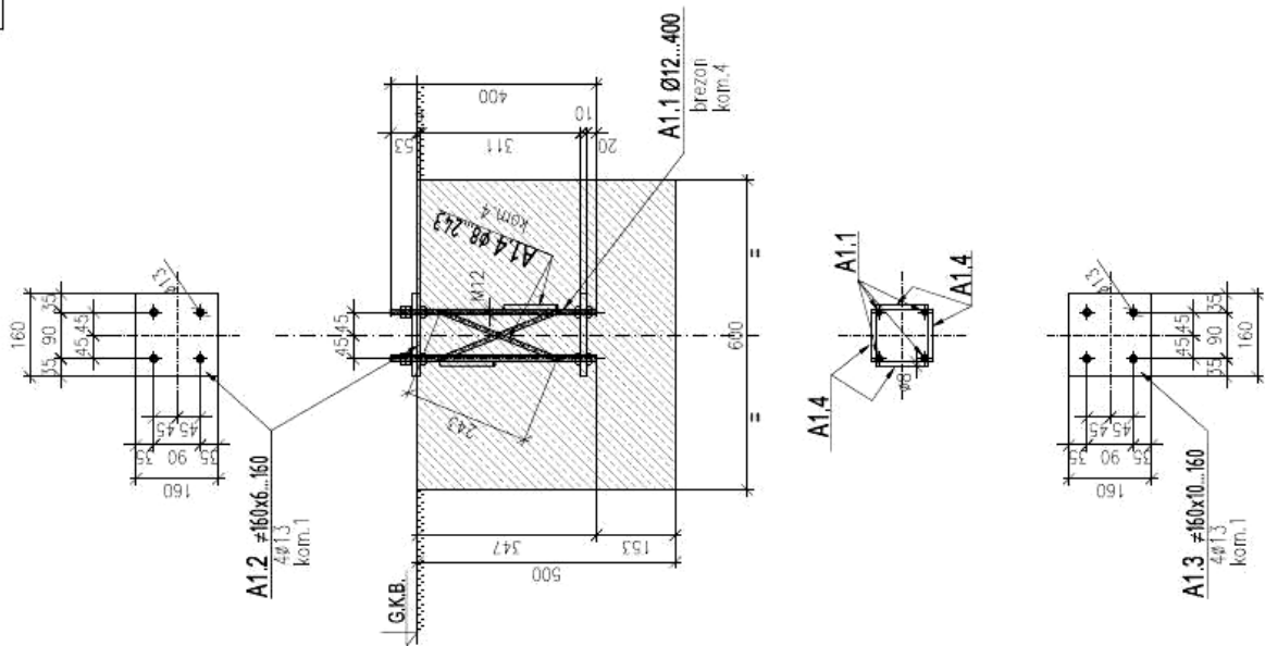
Sl 1: Izgled temeljne stope i ankera za stajališni stub
